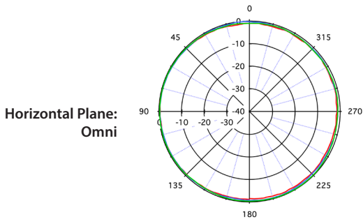
Beamwidth: Horizontal
