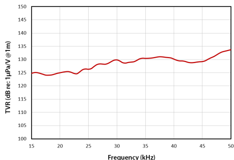
TVR
